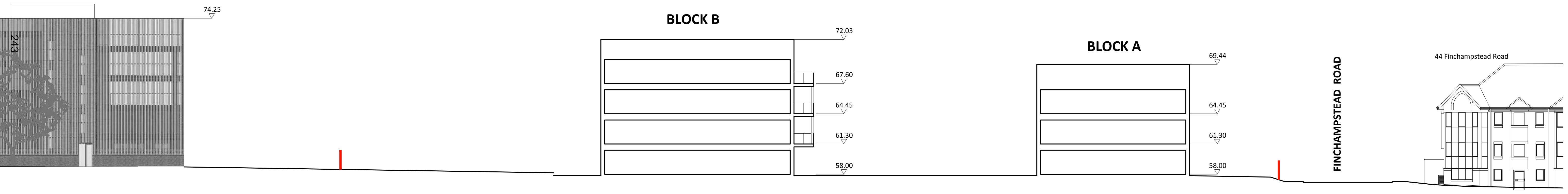
Section BB datum 50.00
